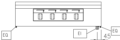
Front aanzicht
