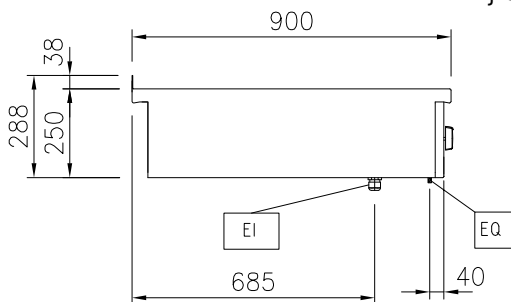
Zij aanzicht
